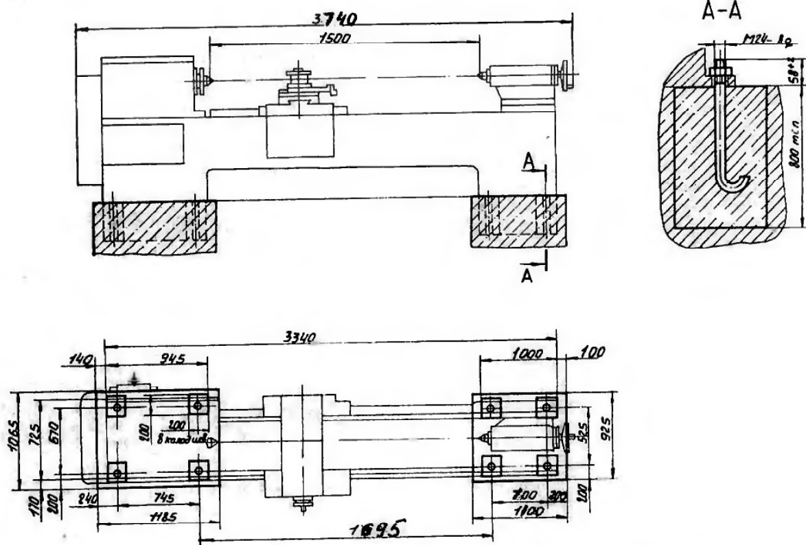
Рис. I.12.2. Монтажный чертеж (фундамент) станка для РМЦ1500.
