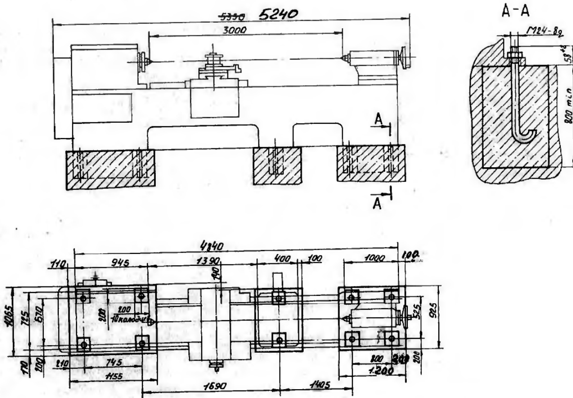
Рис. I.12.3. Монтажный чертеж (фундамент) станка для РМЦ3000.
